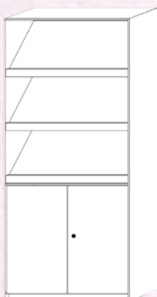
Szafa na czasopisma Nr 96 S-80 G-40 H-180
